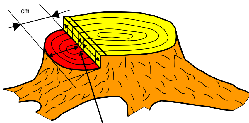
Messstelle in der Mitte der Fallkerbe
